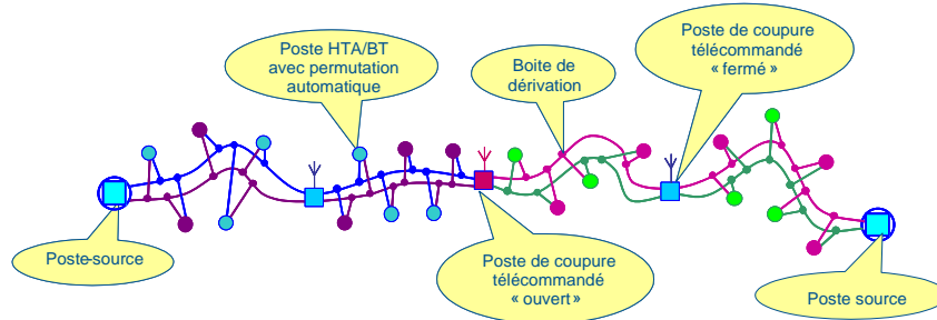
Figure 6 : exemple de structure en double dérivation
