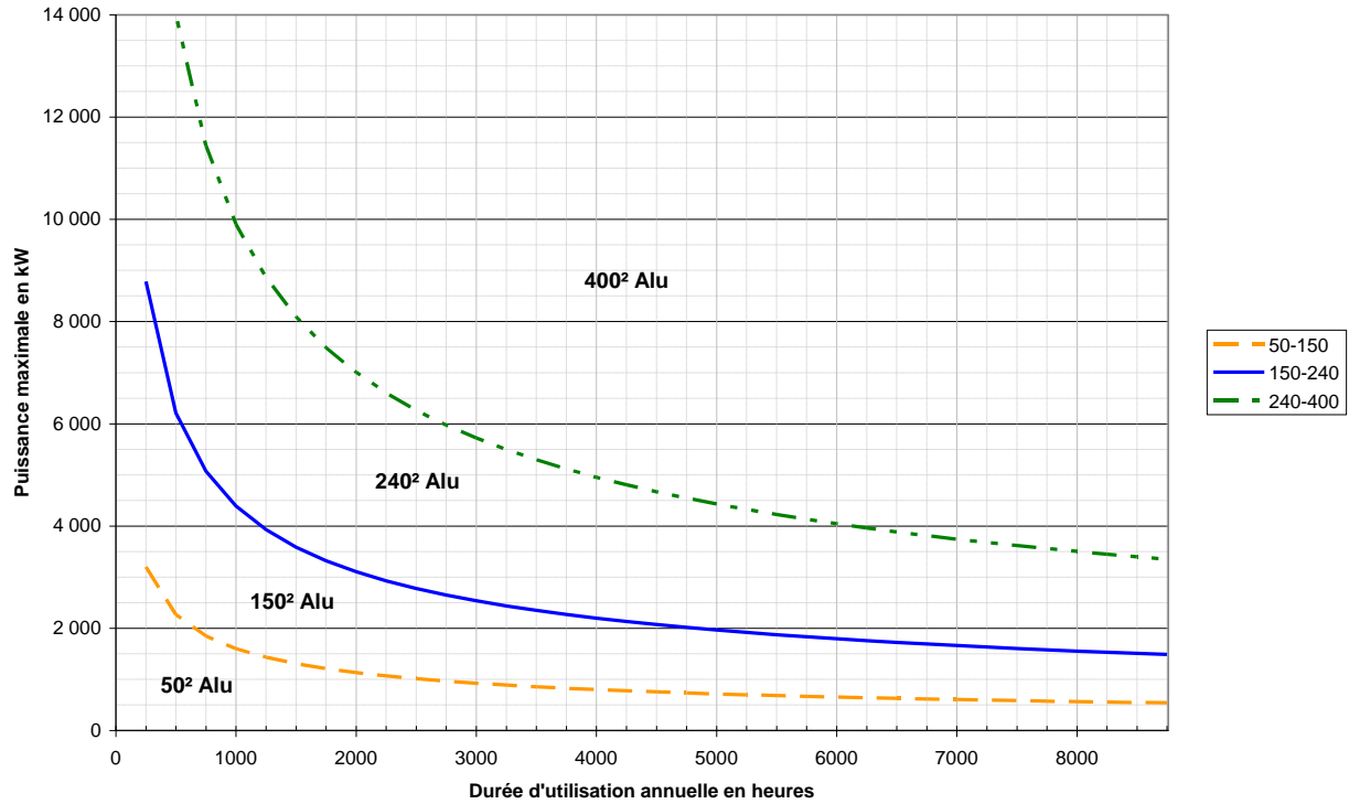
Figure 9 : Abaques des sections économiques de câble (ne prenant pas en compte les intensités admissibles)
