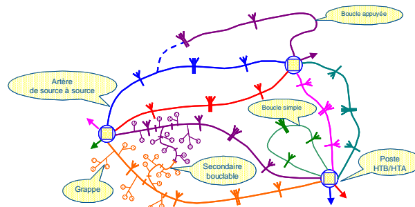
Figure 7 : Structure de réseau rural
